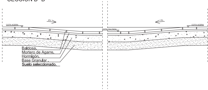
SECCIÓN B-B
