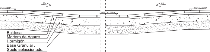
SECCIÓN B-B
