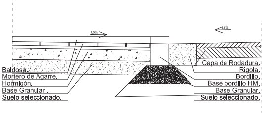
SECCIÓN A-A
